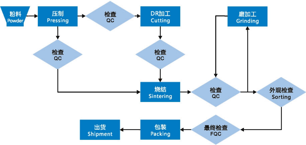
NiZn制造流程图 NiZn Production Flow Diagram
