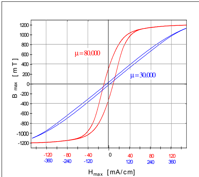
Einstellbare Hysteresen (quasistatisch, 50 Hz)
