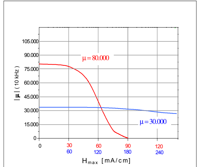
Vormagnetisierungsverhalten
