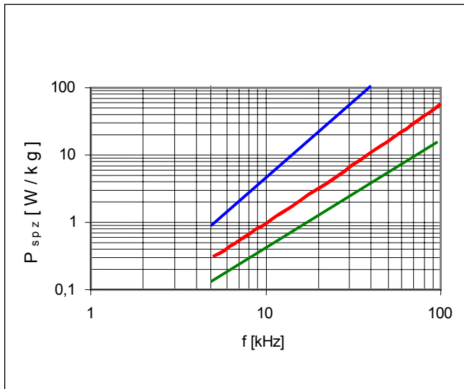
Verluste ( — B = 0,15\text{T} , — B = 0,3\text{T} , — B = 0,6\text{T} )
