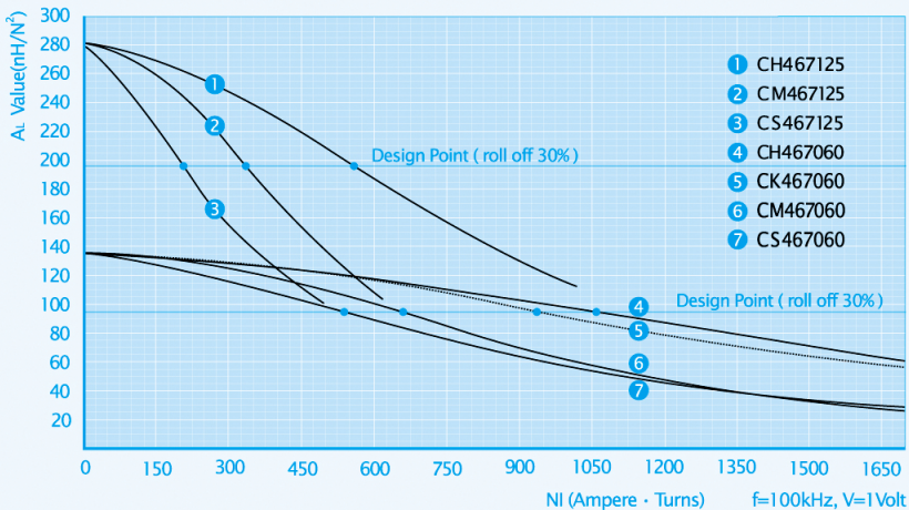
AL vs NI Curve(60μ, 125μ)
